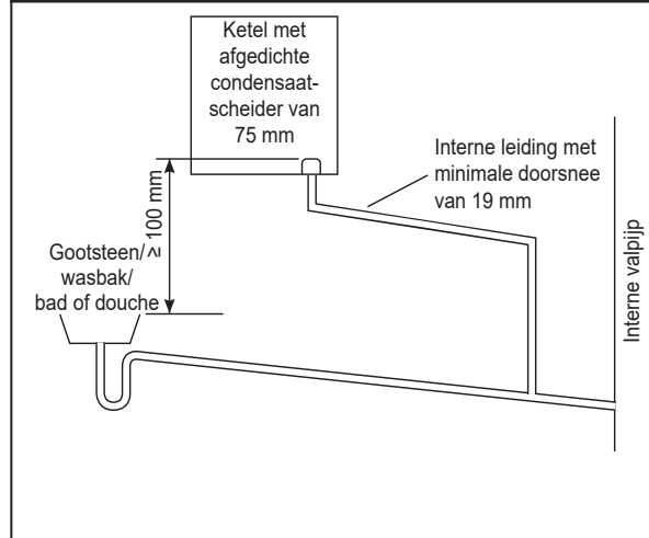
Afbeelding 2 - Aansluiting van de condensatafvoerleiding na de waterscheider van een gootsteen, wastafel, bad of douche op een interne valpijp
