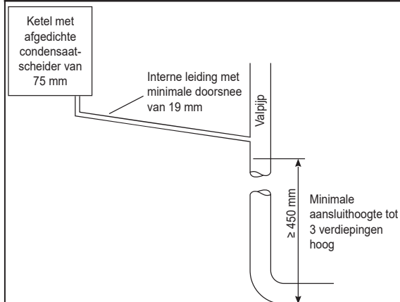
Afbeelding 1 - Aansluiting van de condensatafvoerleiding op een interne valpijp
