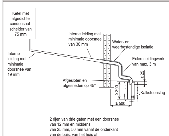
Afbeelding 6 - Aansluiting van de condensatafvoerleiding op een extern, speciaal ontworpen wegsijpelpunt.
