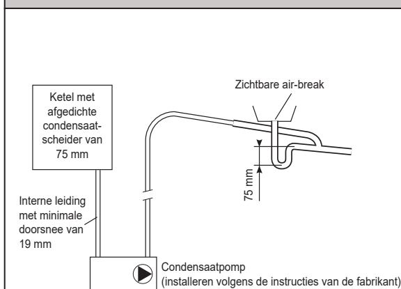
Afbeelding 3 - Typische aansluiting van de condensaatpomp (raadpleeg de uitgebreide aanwijzingen van de fabrikant)
