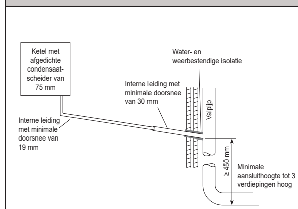
Afbeelding 4 - Aansluiting van de condensatafvoerleiding op een externe valpijp
