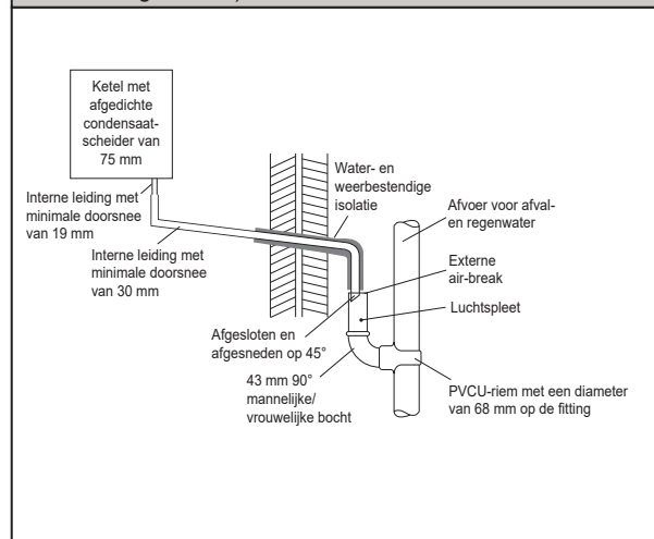
Afbeelding 5 - Aansluiting van de condensatafvoerleiding op een externe regenwaterpijp (alleen een afvoer voor afval- en regenwater)
